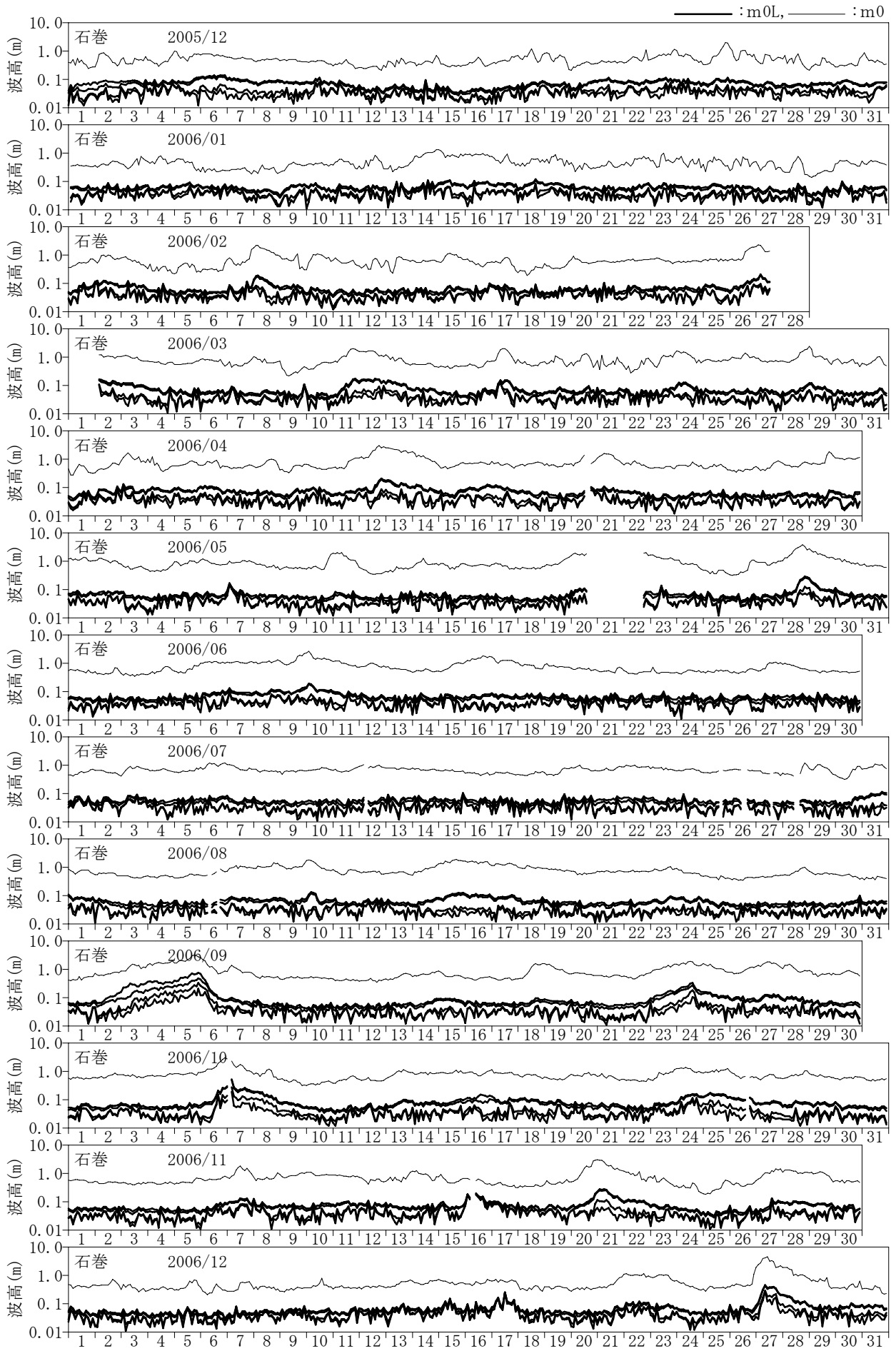
付図-C.1.35 長周期波高の経時変化図 (石巻)
