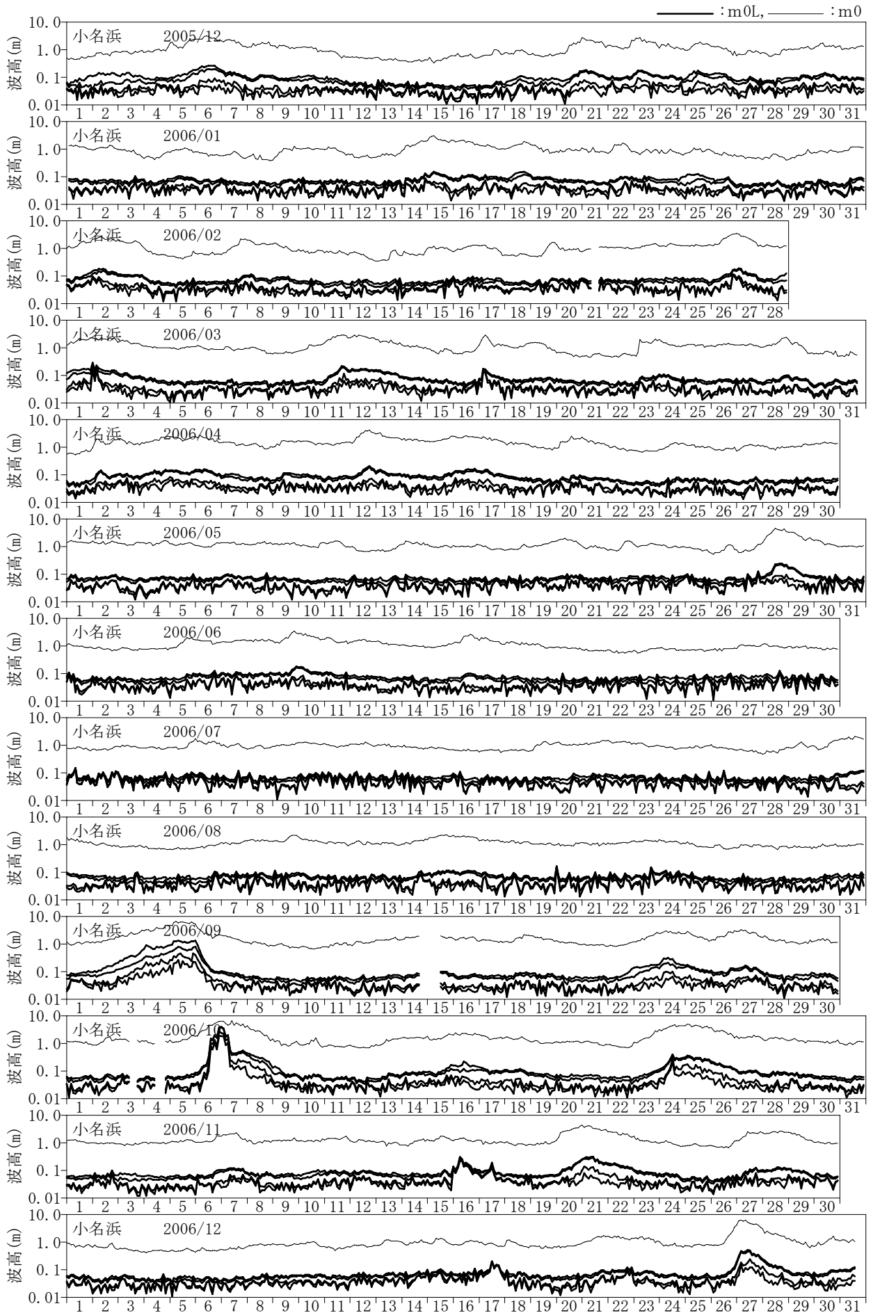
付図-C.1.38 長周期波高の経時変化図 (小名浜)
