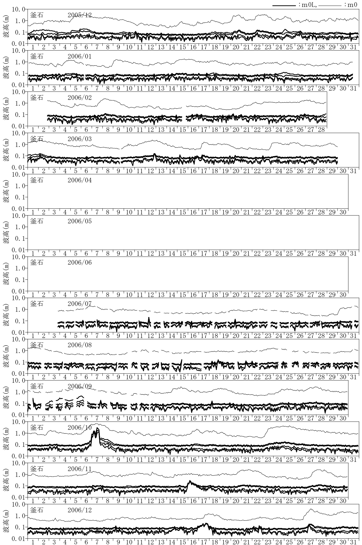
付図-C.1.34 長周期波高の経時変化図 (釜石)
