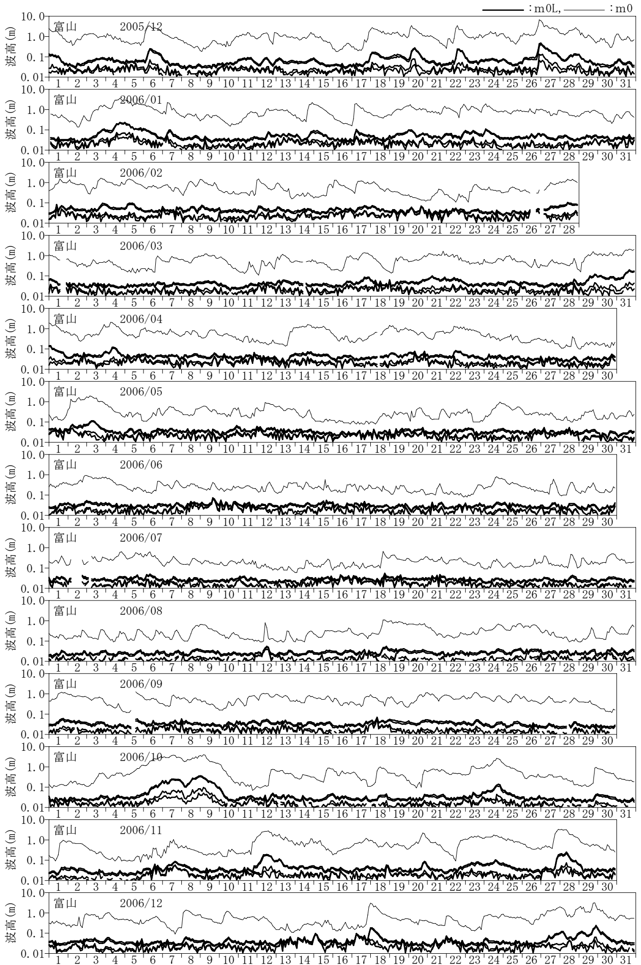
付図-C.1.10 長周期波高の経時変化図 (富山)
