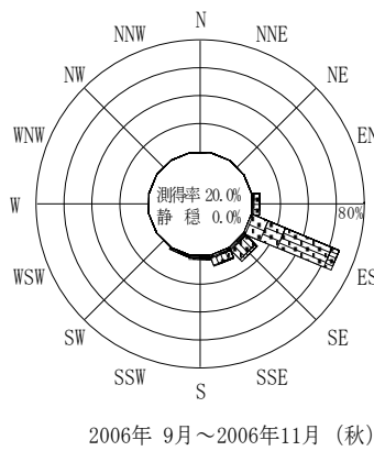
付図-B.2.56 細島 波高・波向別出現頻度図（連続観測）
