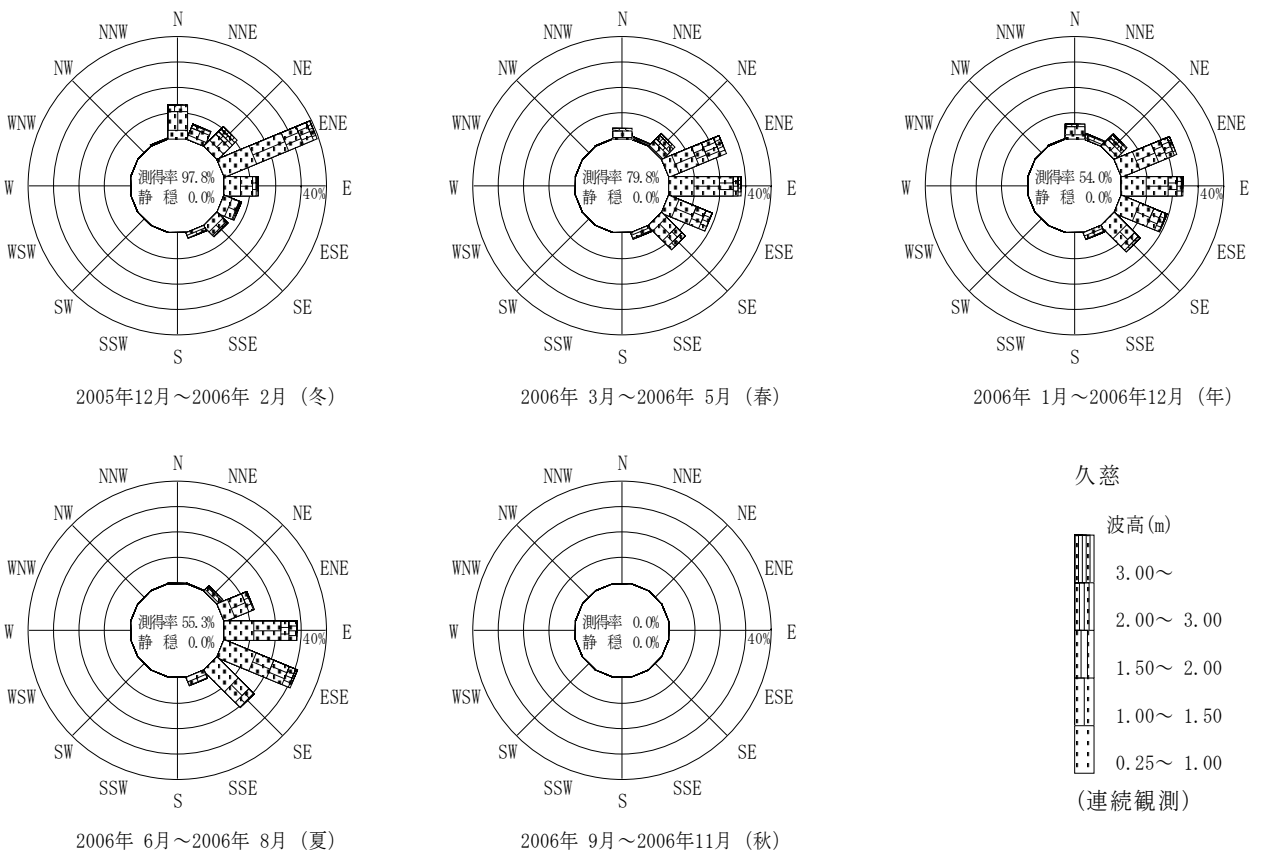
付図-B.2.33 久慈 波高・波向別出現頻度図（連続観測）
