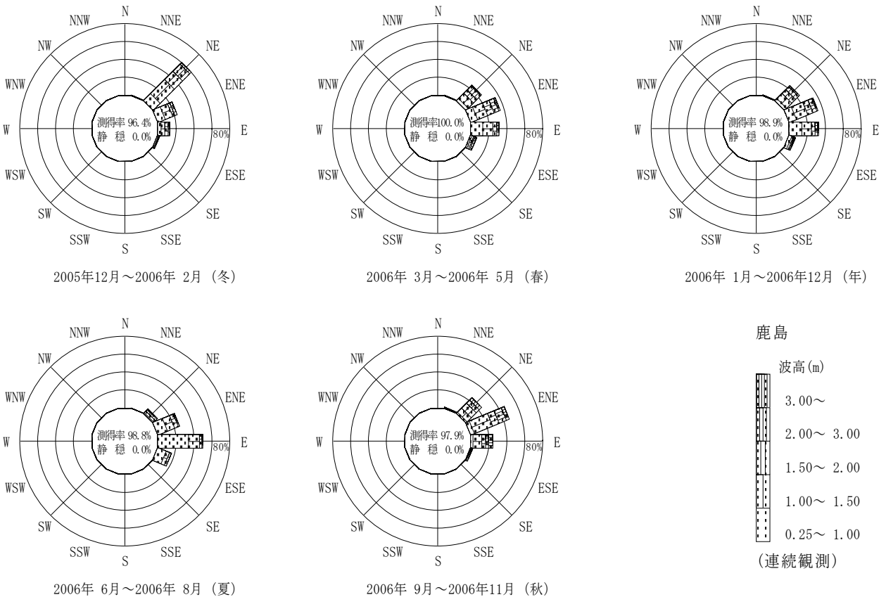
付図-B.2.40 鹿島 波高・波向別出現頻度図（連続観測）
