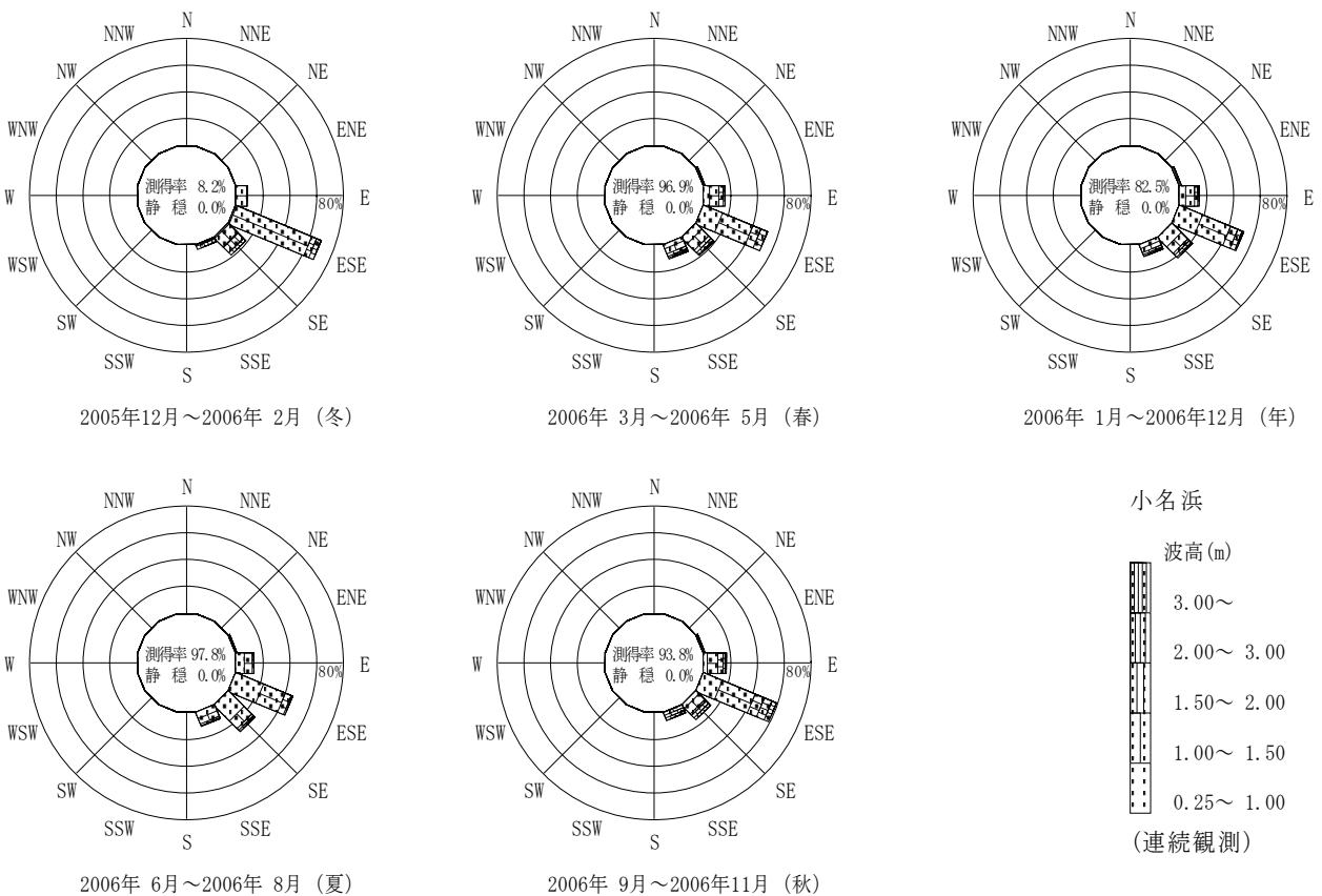
付図-B.2.38 小名浜 波高・波向別出現頻度図（連続観測）
