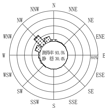
付図-A.2.62 石垣沖 波高・波向別出現頻度図
