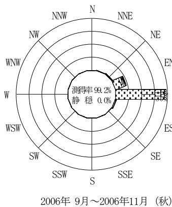
付図-A. 2. 32 八戸 波高・波向別出現頻度図
