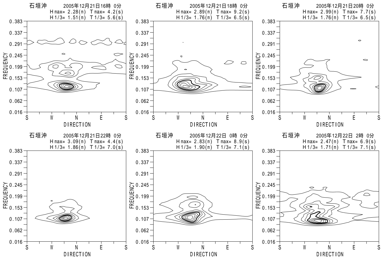
付図 - A.5.61 石垣沖 代表的な高波期間中の方向スペクトル
