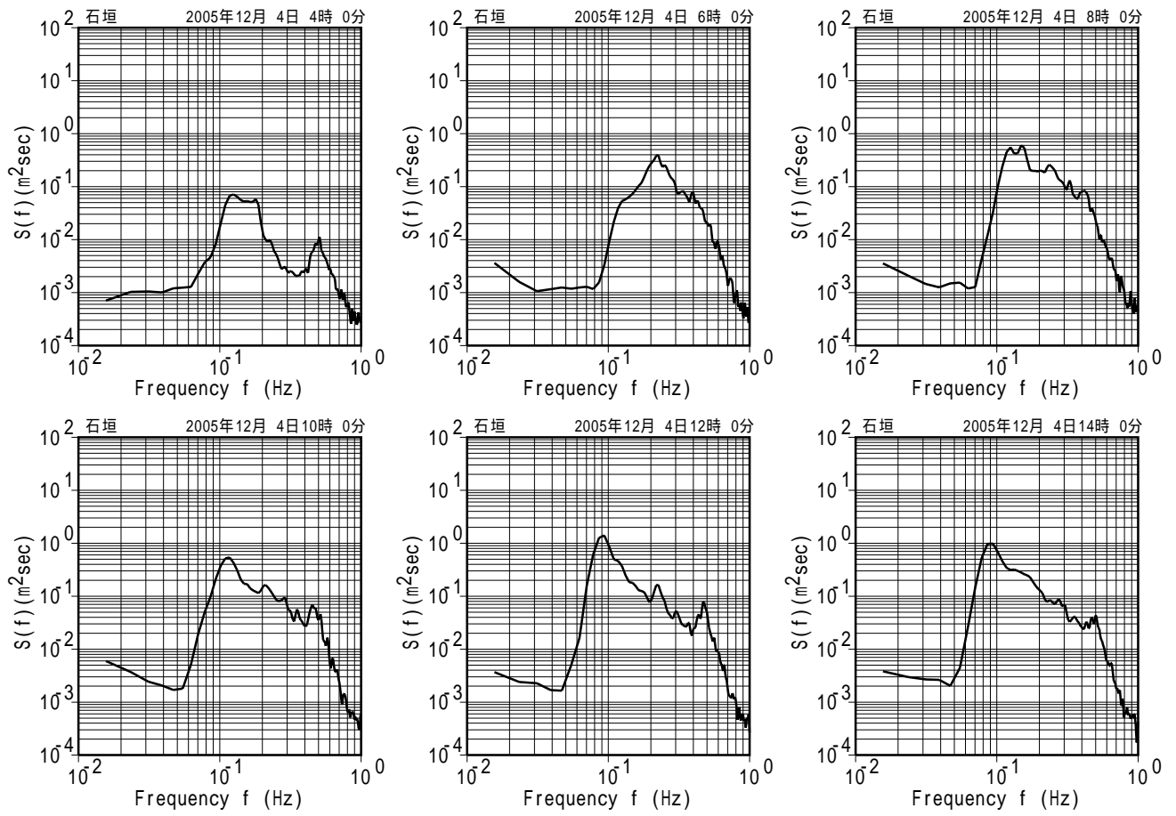
付図 - A.5.60 石垣 代表的な高波期間中のスペクトル
