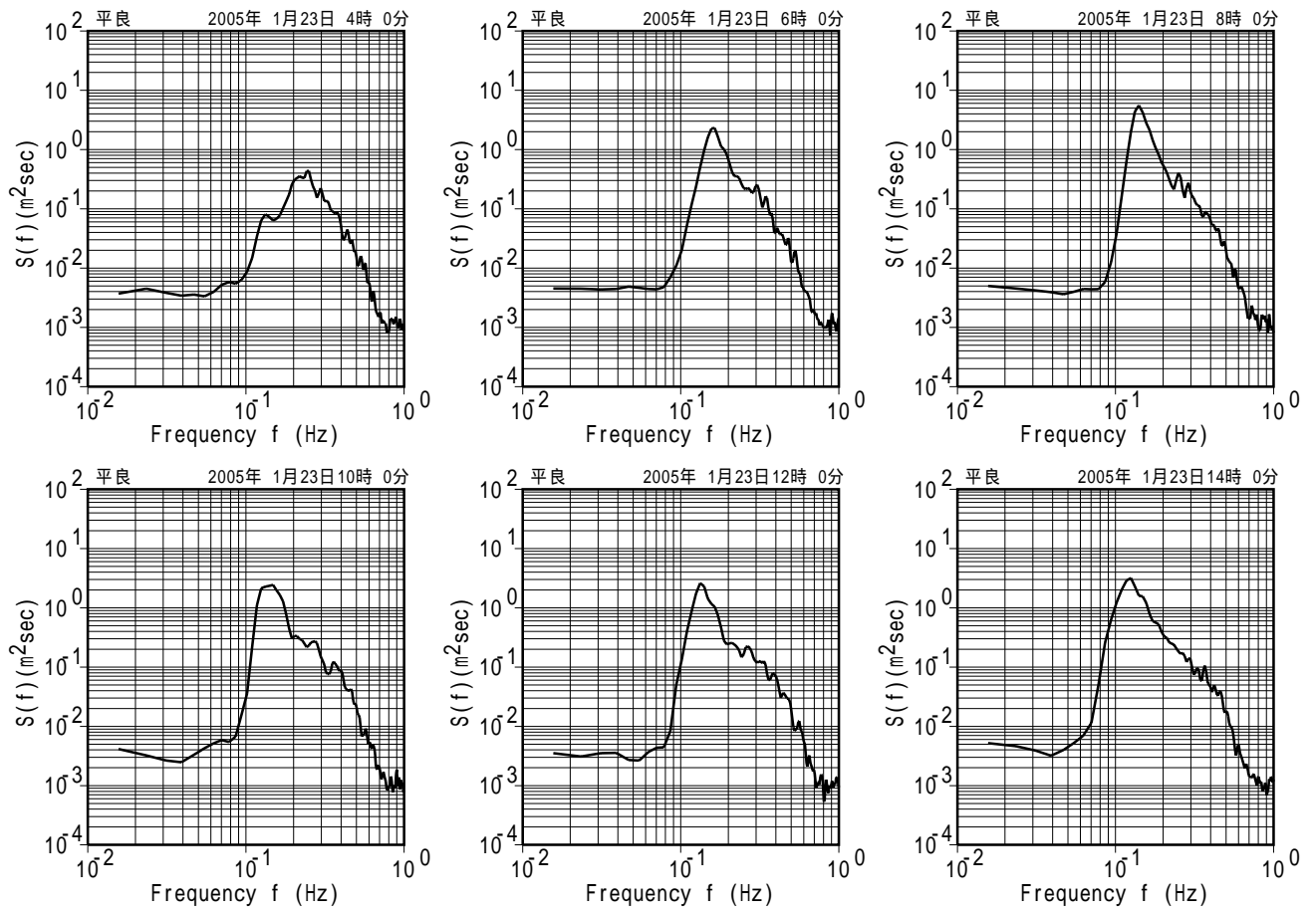
付図 - A.5.58 平良 代表的な高波期間中のスペクトル
