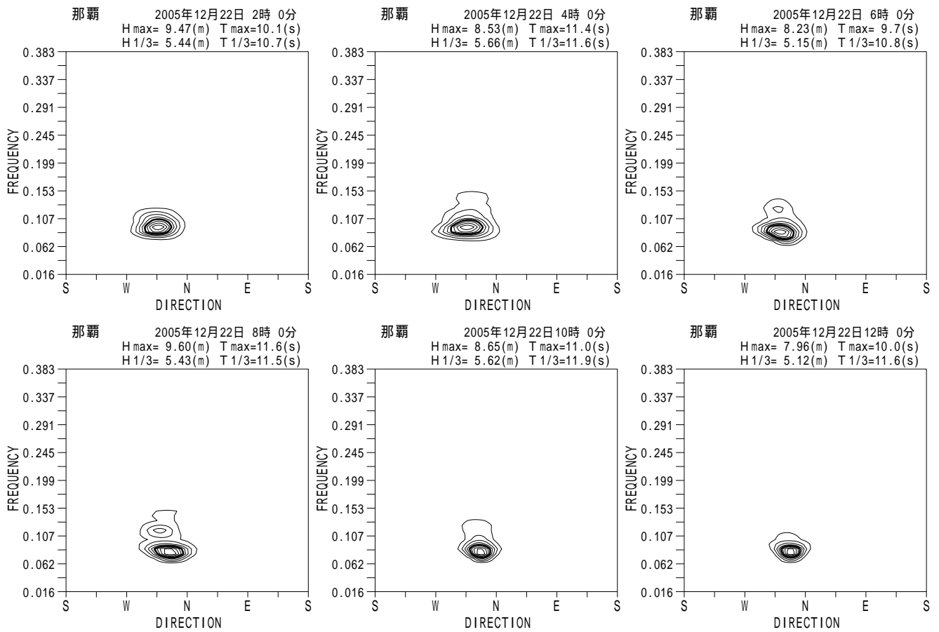
付図 - A.5.24 那覇 代表的な高波期間中の方向スペクトル
