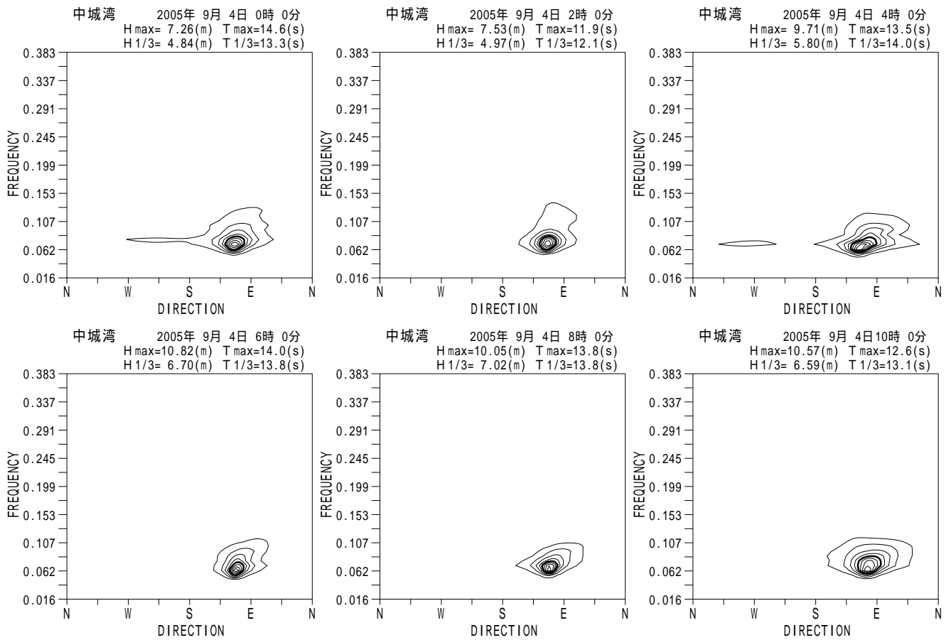
付図 - A.5.57 中城湾 代表的な高波期間中の方向スペクトル
