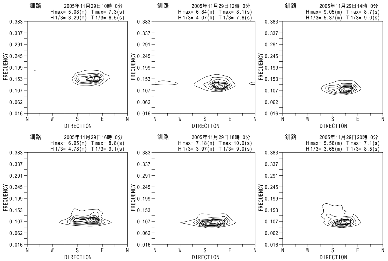
付図 - A.5.26 釧路 代表的な高波期間中の方向スペクトル
