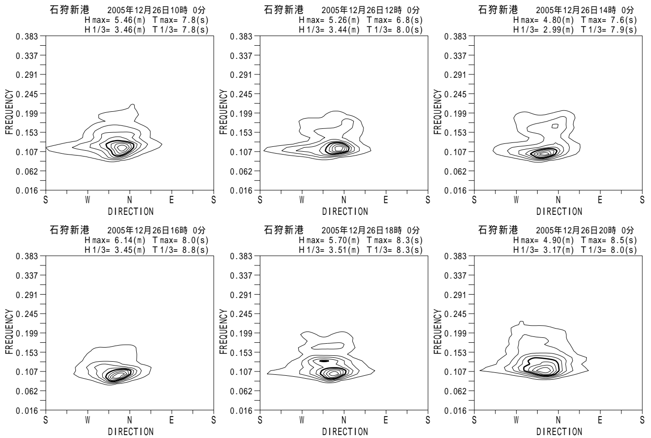
付図 - A.5.2 石狩新港 代表的な高波期間中の方向スペクトル
