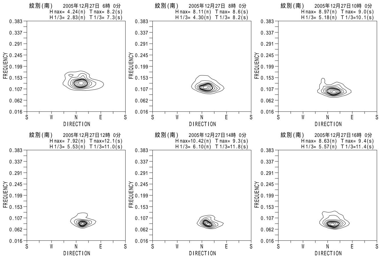
付図 - A.5.25 紋別(南) 代表的な高波期間中の方向スペクトル
