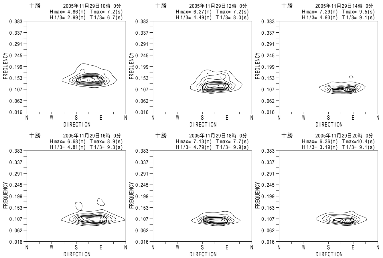
付図 - A.5.27 十勝 代表的な高波期間中の方向スペクトル
