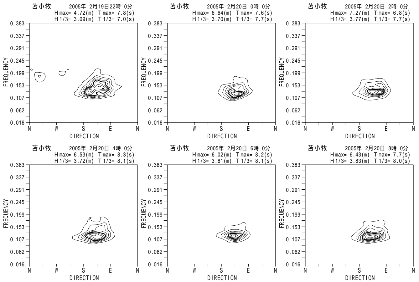
付図 - A.5.28 苦小牧 代表的な高波期間中の方向スペクトル
