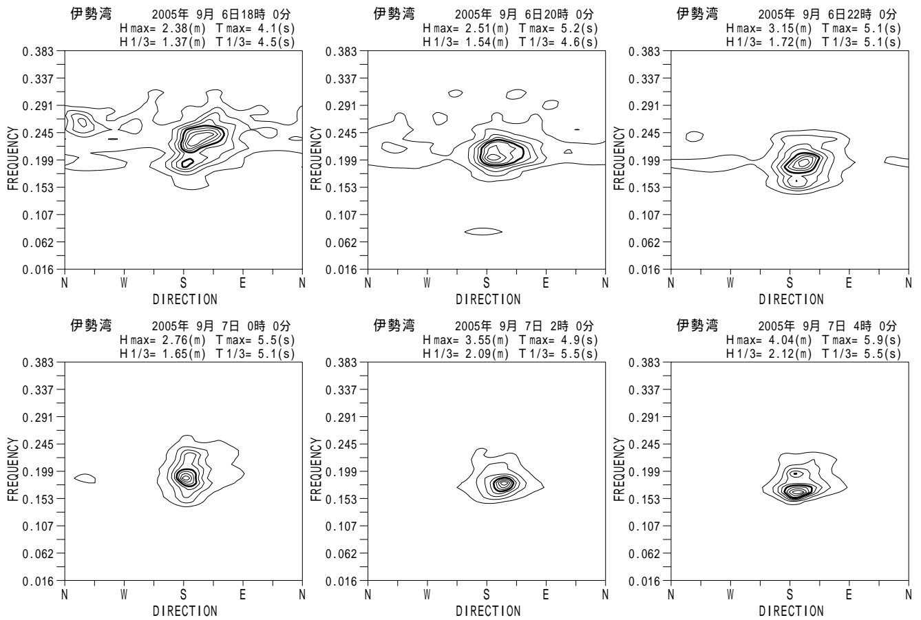
付図 - A.5.45 伊勢湾 代表的な高波期間中の方向スペクトル
