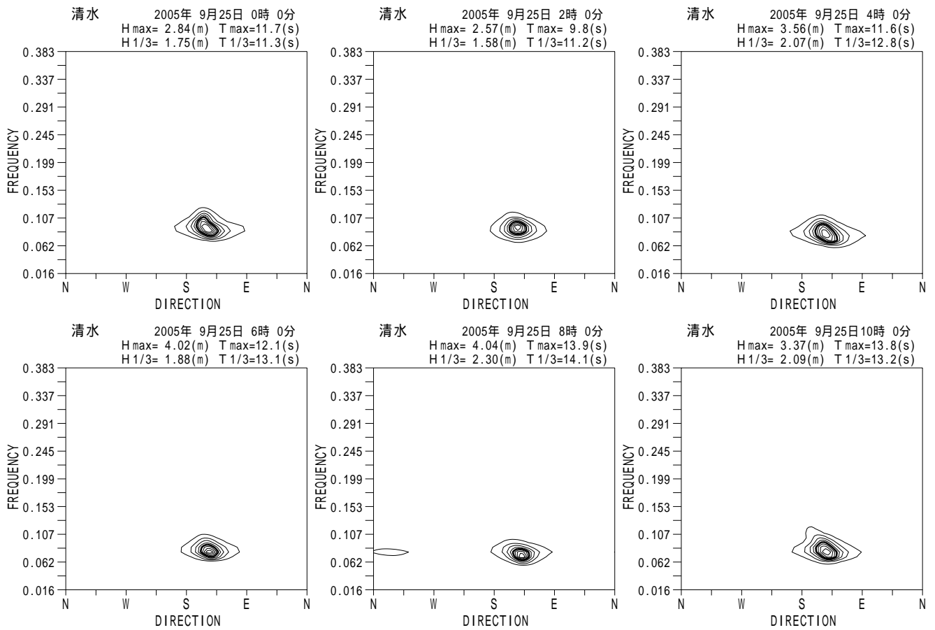
付図 - A.5.43 清水 代表的な高波期間中の方向スペクトル
