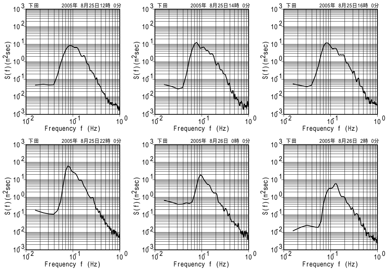
付図 - A.5.42 下田 代表的な高波期間中のスペクトル
