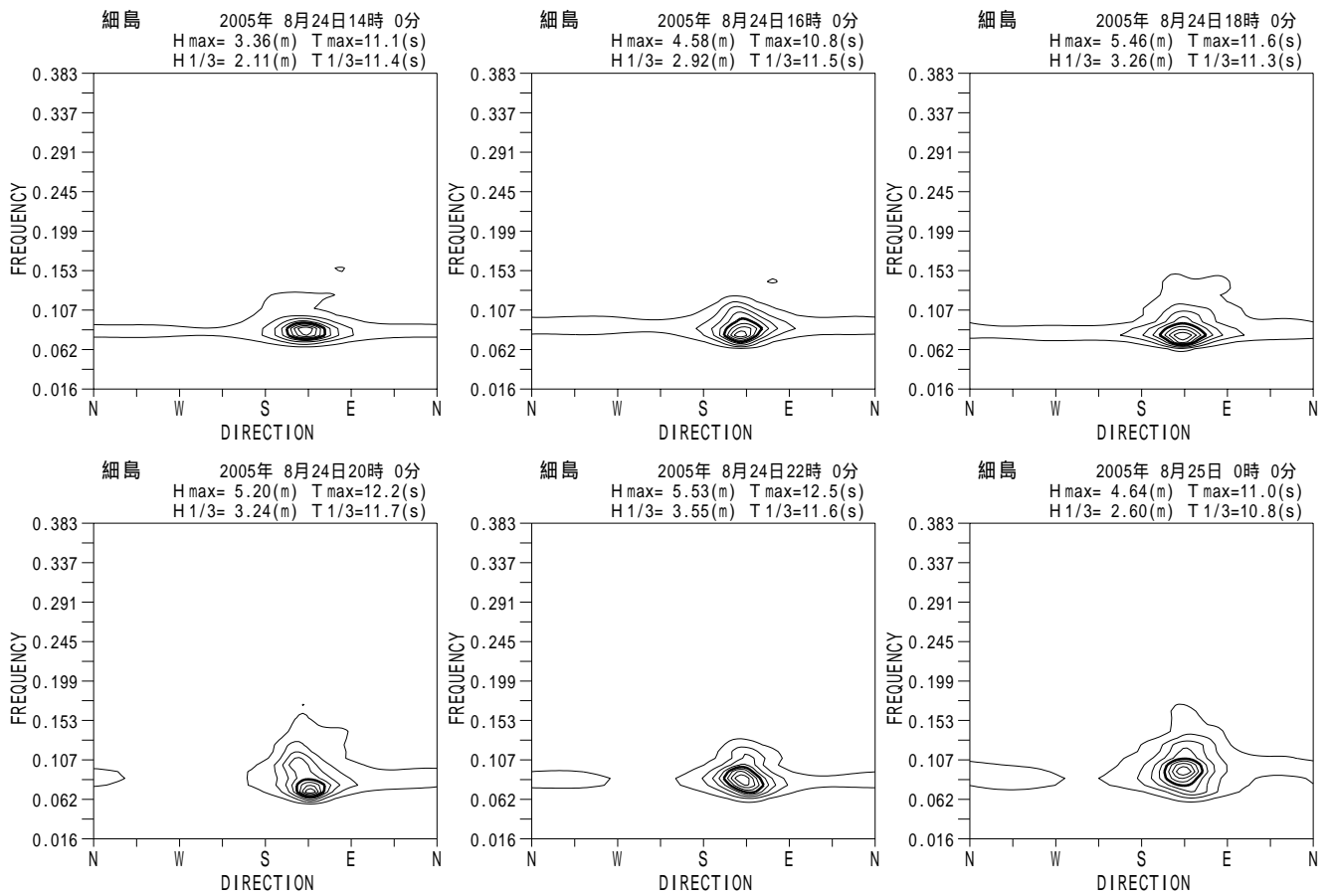
付図 - A.5.54 細島 代表的な高波期間中の方向スペクトル
