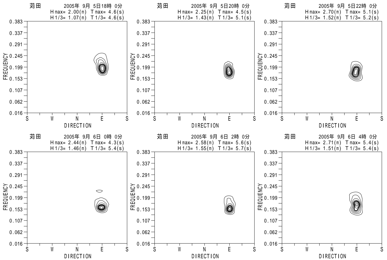
付図 - A.5.53 苅田 代表的な高波期間中の方向スペクトル
