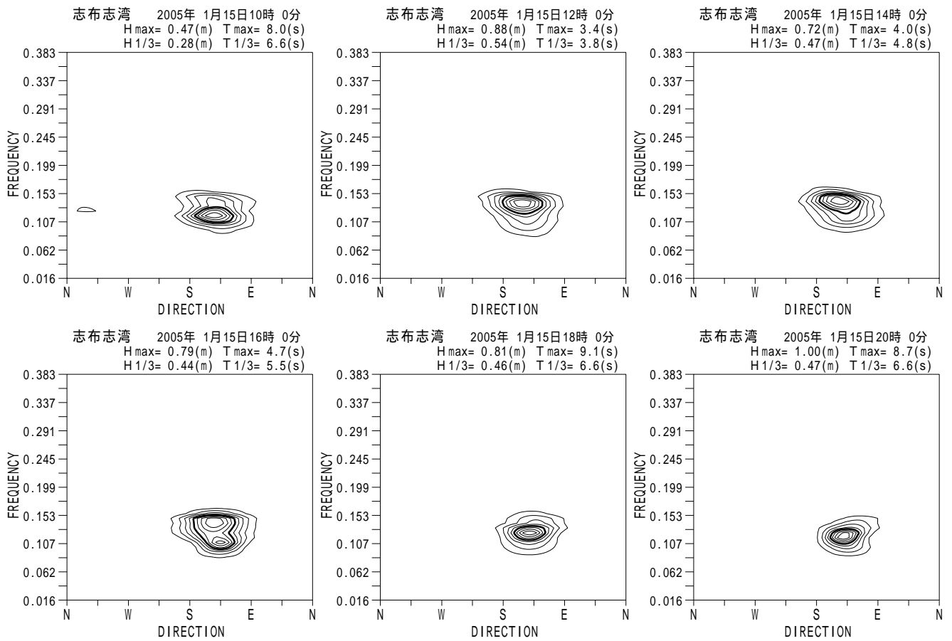
付図 - A.5.55 志布志湾 代表的な高波期間中の方向スペクトル
