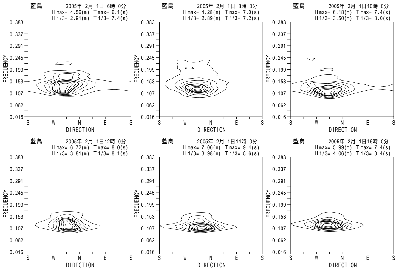
付図 - A.5.20 藍島 代表的な高波期間中の方向スペクトル
