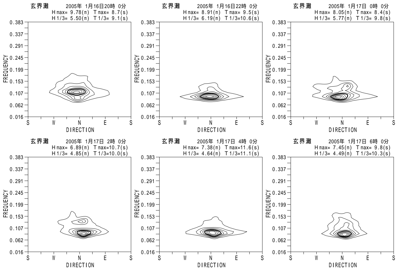
付図 - A.5.21 玄界灘 代表的な高波期間中の方向スペクトル
