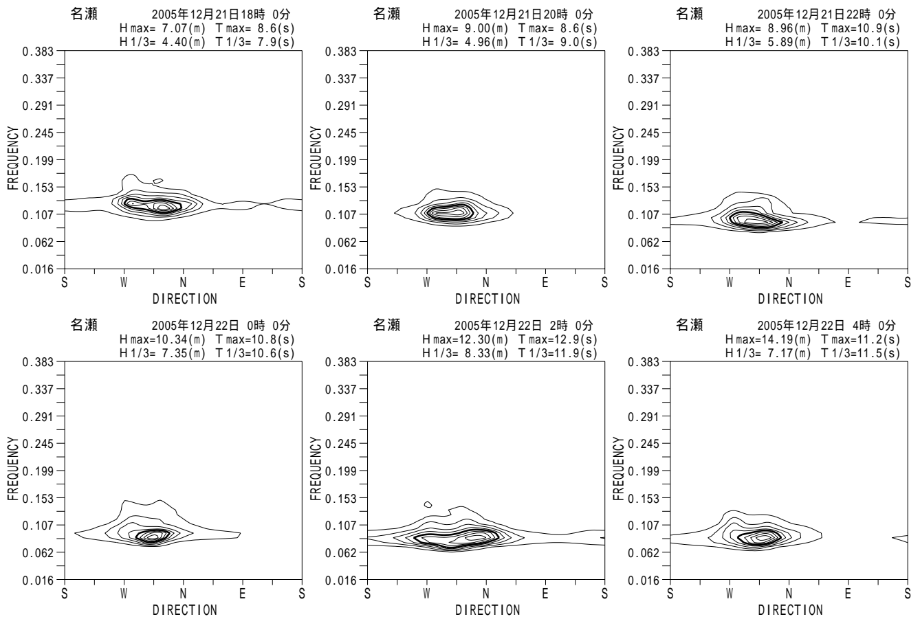
付図 - A.5.23 名瀬 代表的な高波期間中の方向スペクトル
