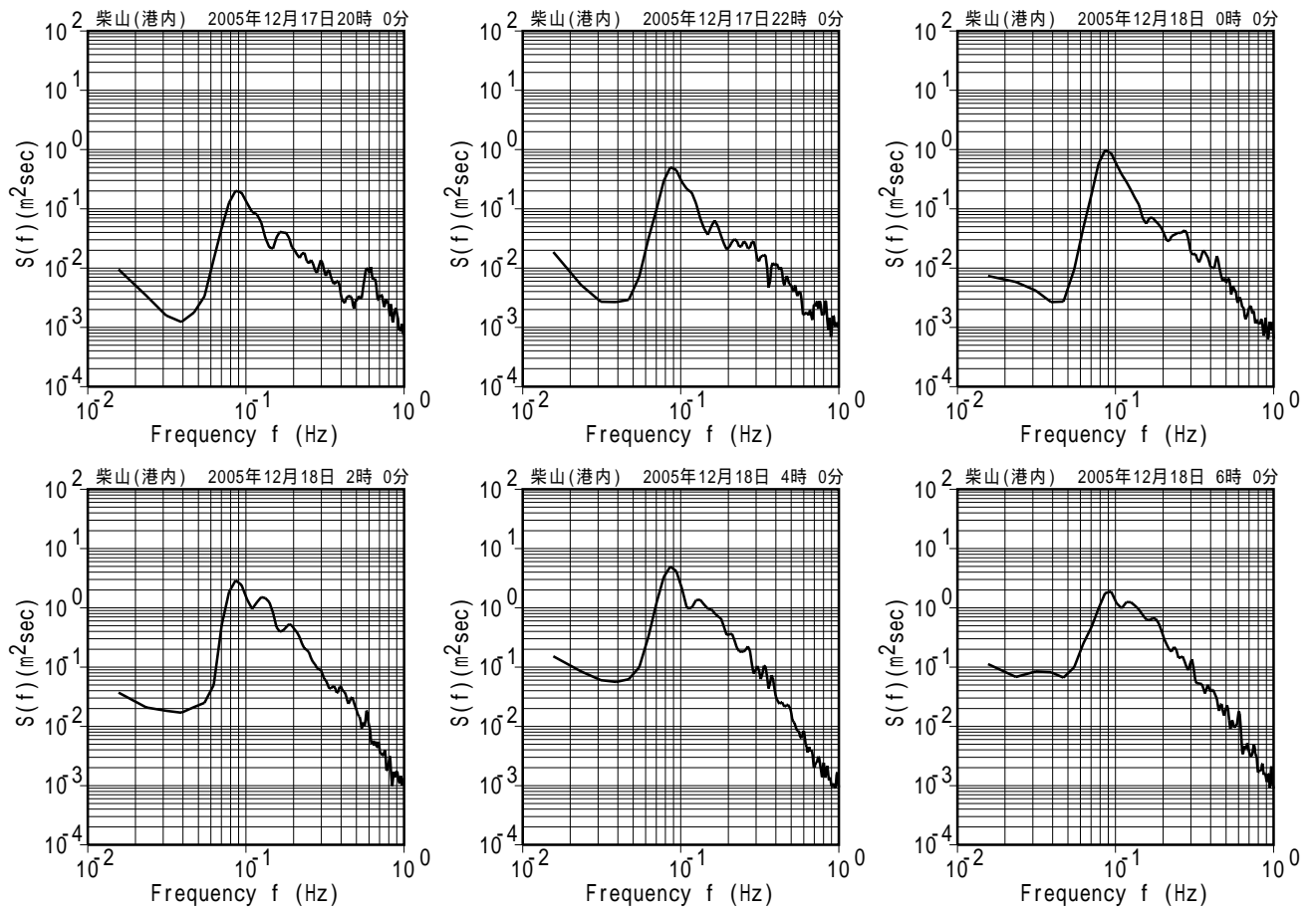
付図 - A.5.16 柴山(港内) 代表的な高波期間中のスペクトル
