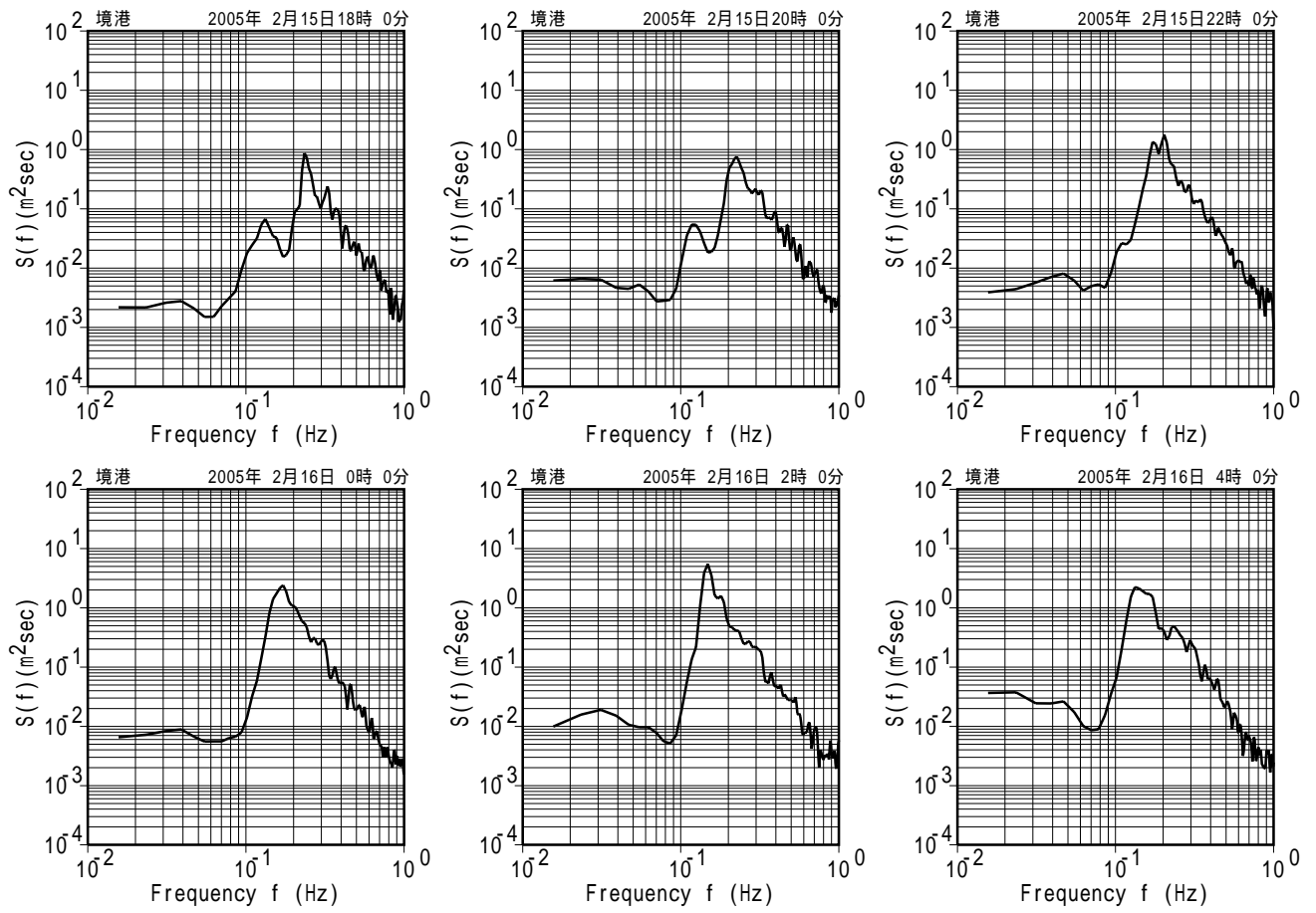
付図 - A.5.18 境港 代表的な高波期間中のスペクトル
