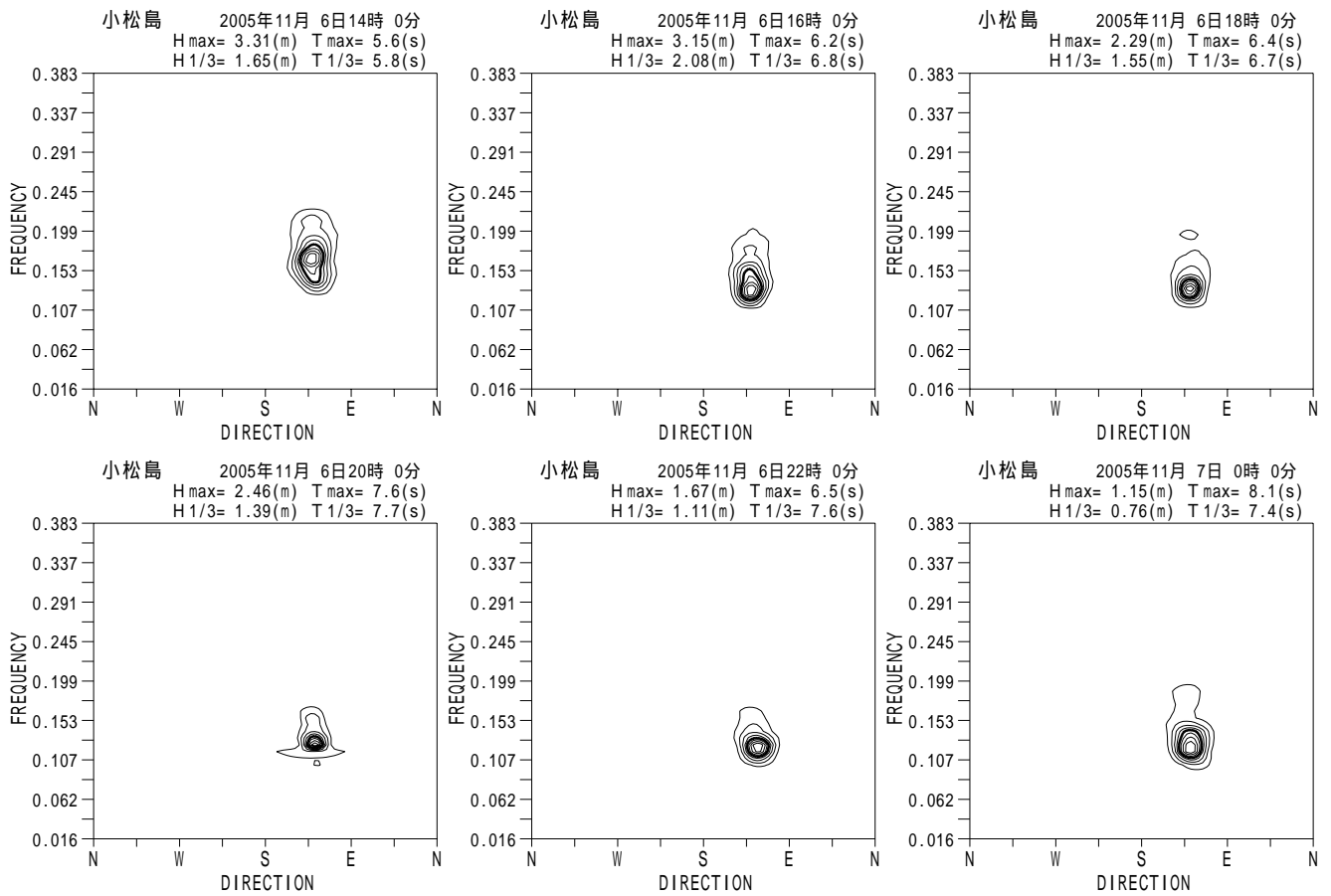
付図 - A.5.48 小松島 代表的な高波期間中の方向スペクトル
