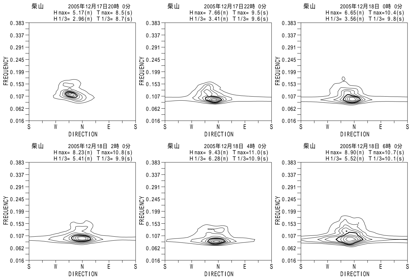
付図 - A.5.15 柴山 代表的な高波期間中の方向スペクトル
