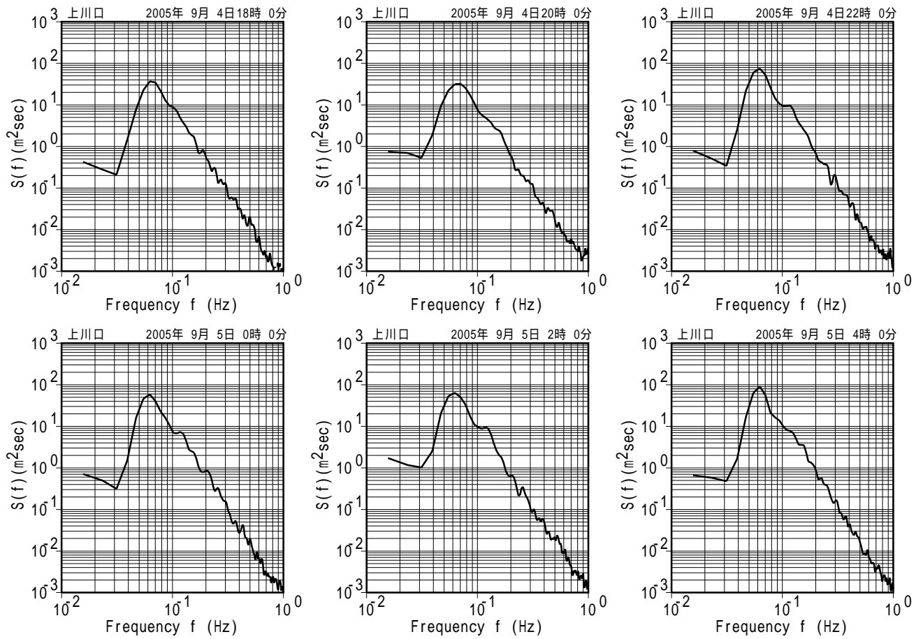
付図 - A.5.52 上川口 代表的な高波期間中のスペクトル
