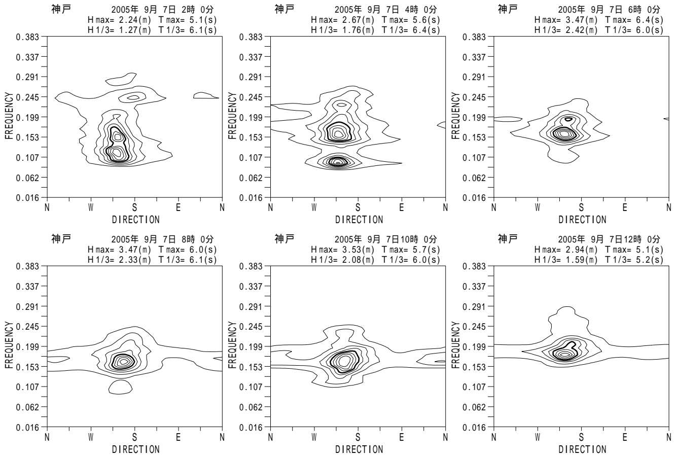
付図 - A.5.47 神戸 代表的な高波期間中の方向スペクトル
