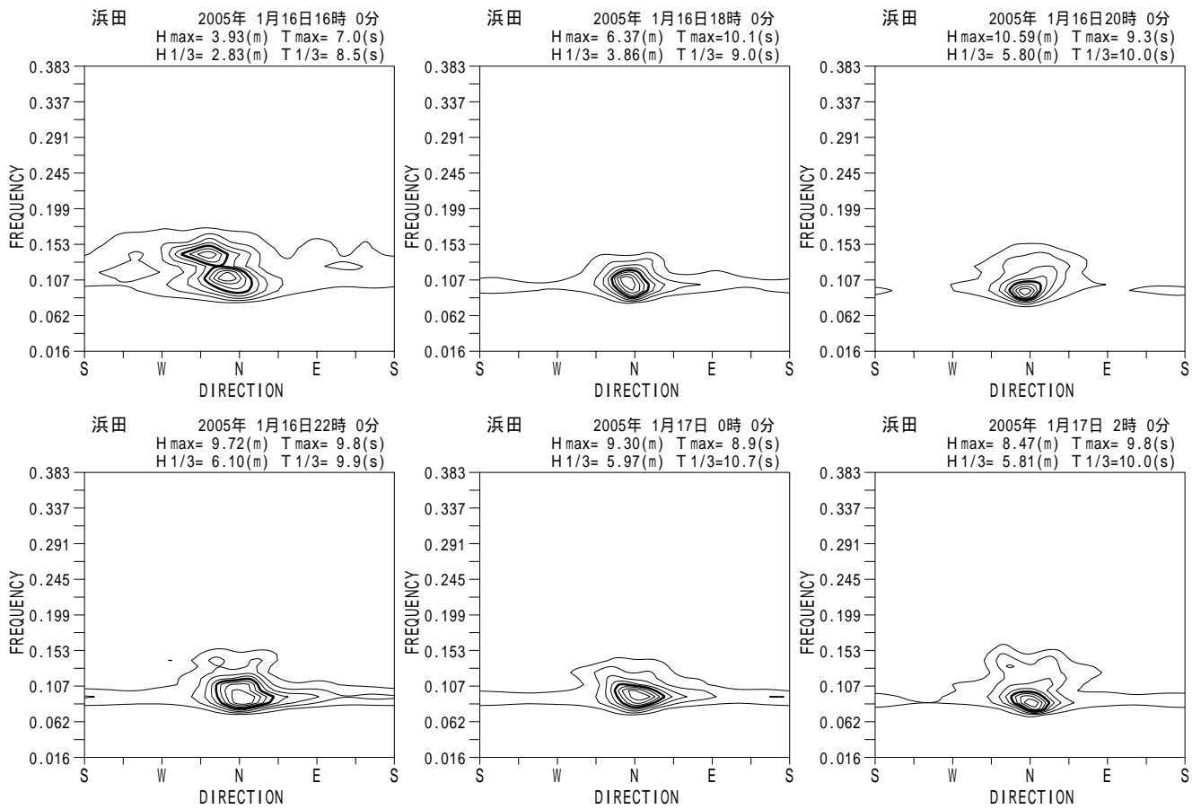
付図 - A.5.19 浜田 代表的な高波期間中の方向スペクトル
