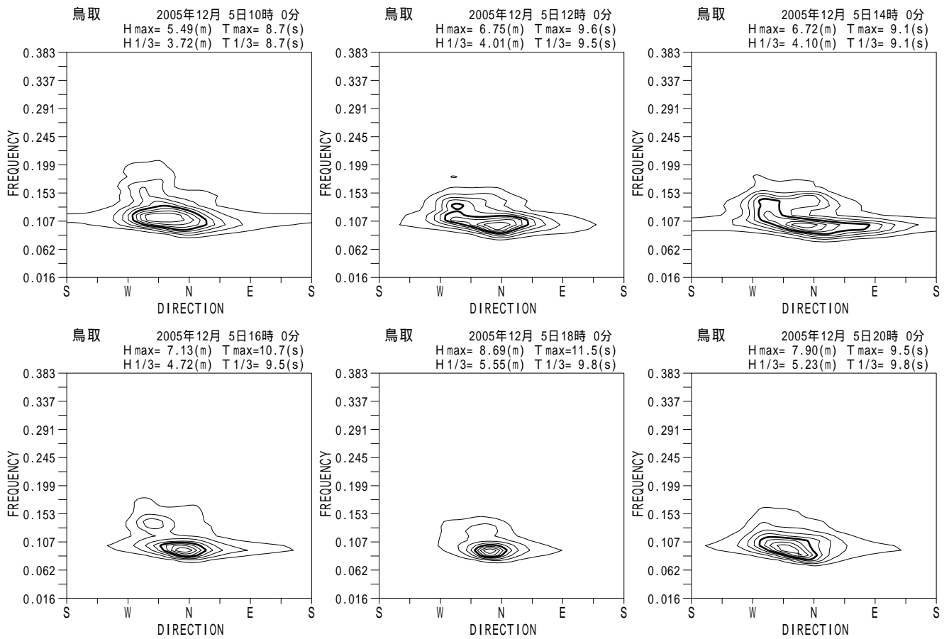
付図 - A.5.17 鳥取 代表的な高波期間中の方向スペクトル
