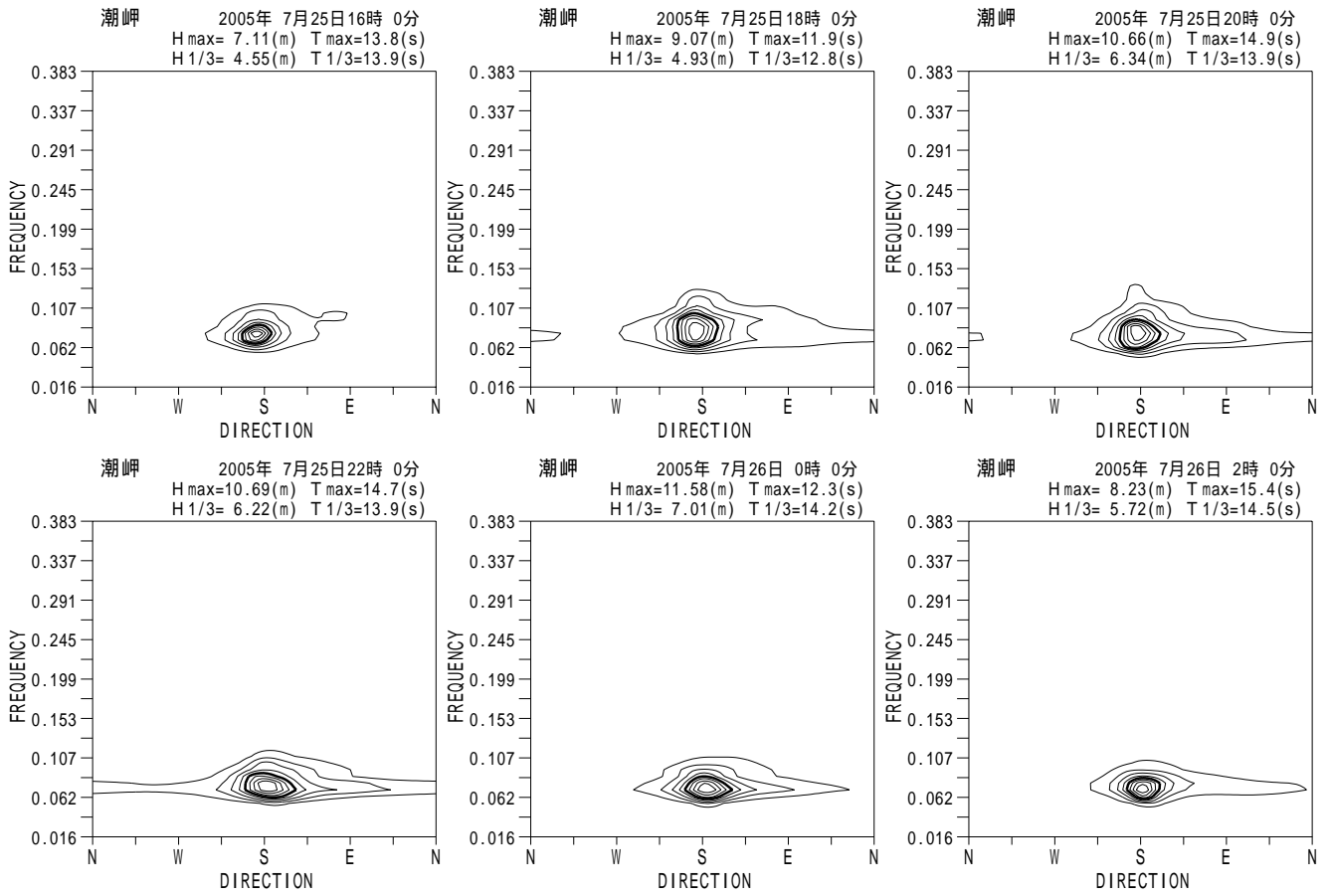
付図 - A.5.46 潮岬 代表的な高波期間中の方向スペクトル
