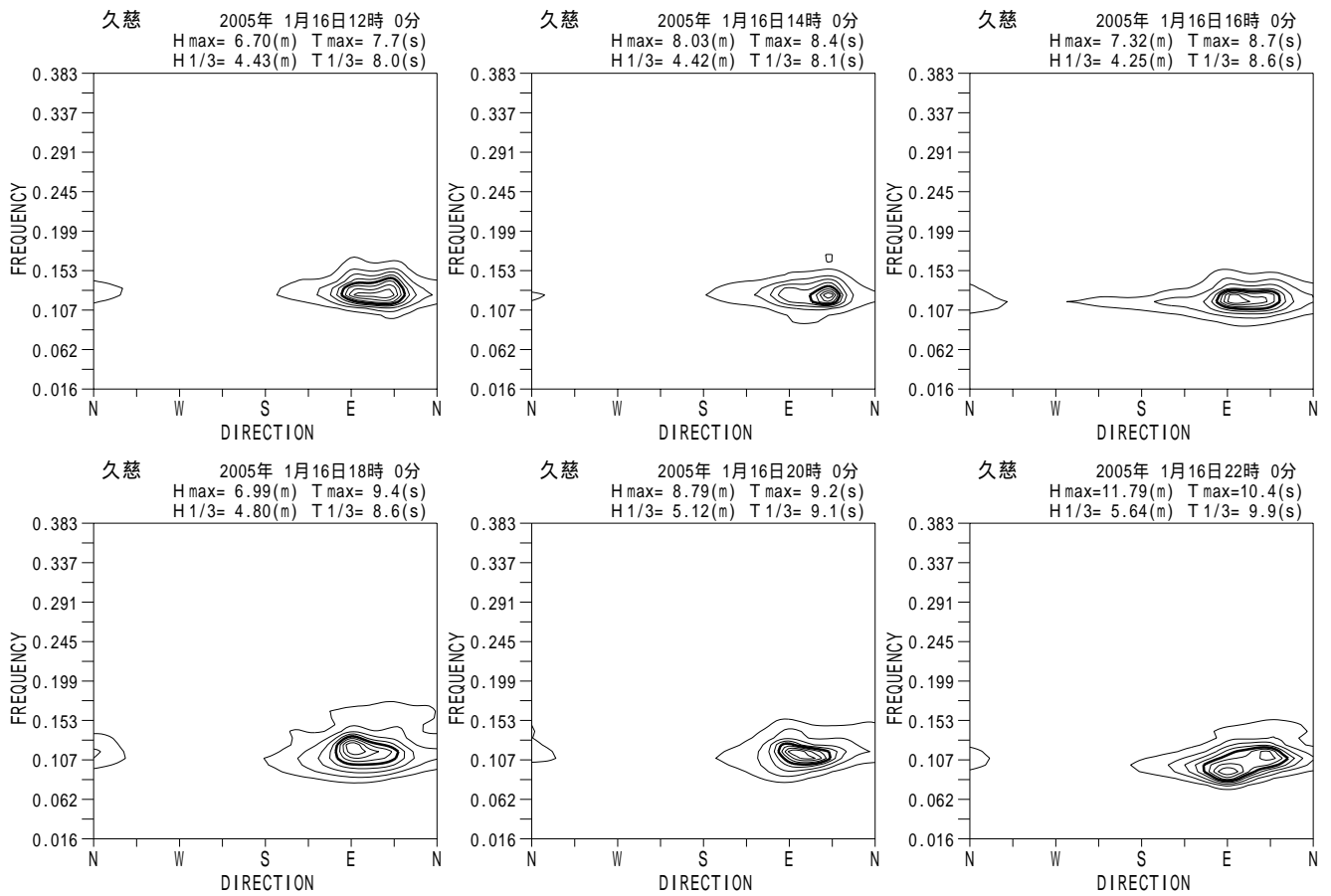
付図 - A.5.31 久慈 代表的な高波期間中の方向スペクトル
