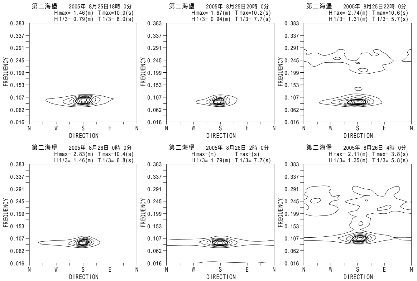
付図 - A.5.39 第二海堡 代表的な高波期間中の方向スペクトル
