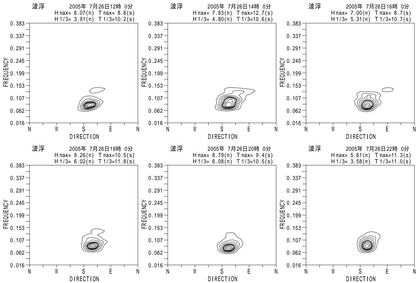
付図 - A.5.41 波浮 代表的な高波期間中の方向スペクトル
