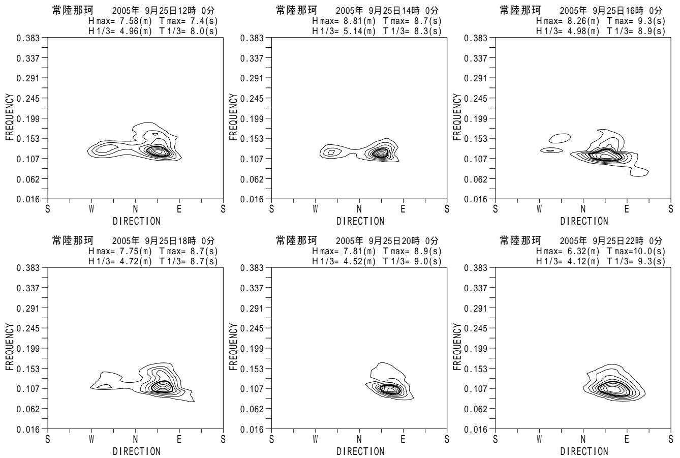
付図 - A.5.37 常陸那珂 代表的な高波期間中の方向スペクトル
