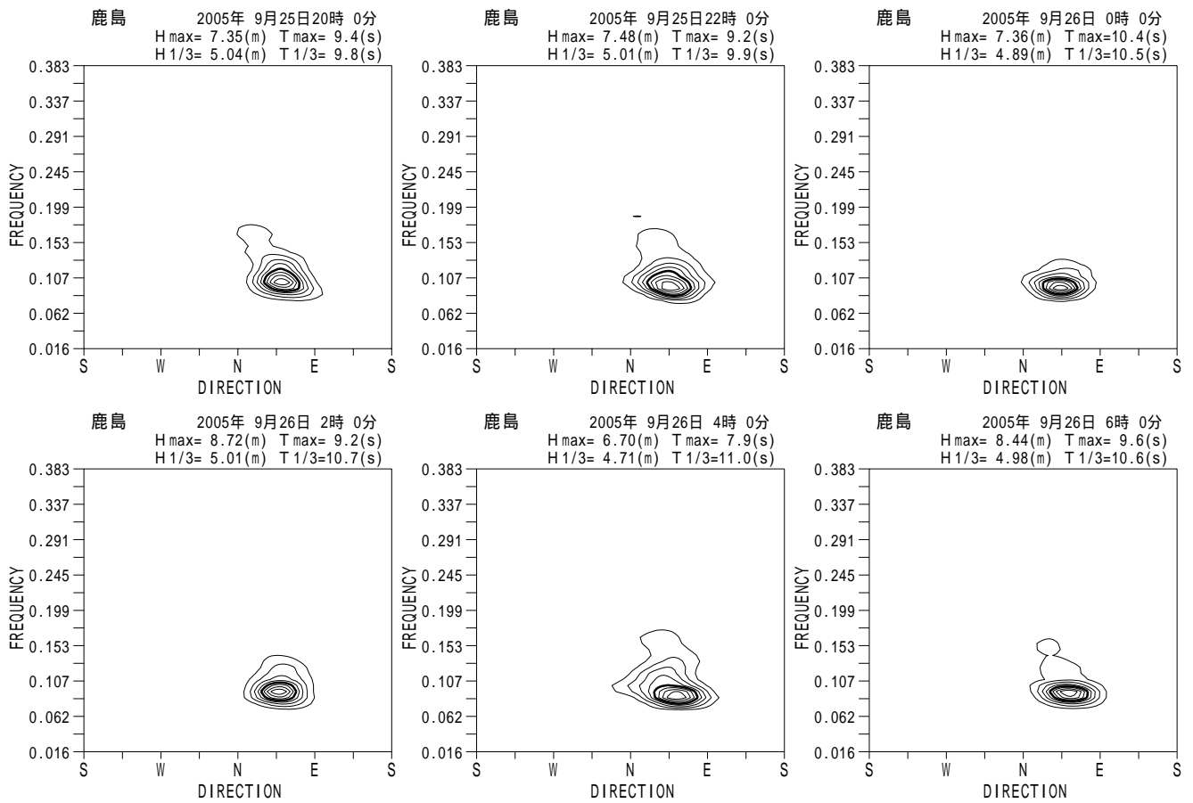
付図 - A.5.38 鹿島 代表的な高波期間中の方向スペクトル
