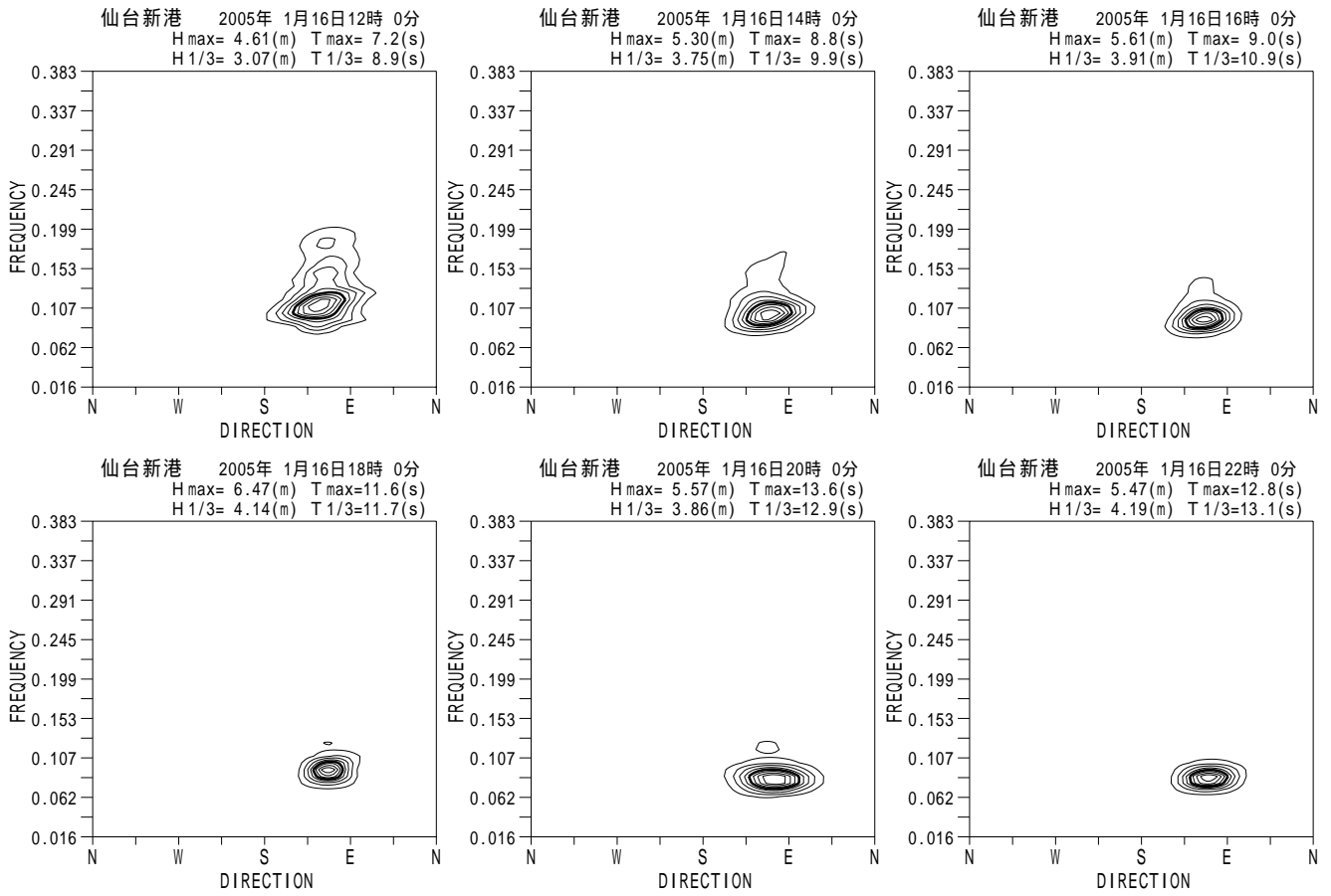
付図 - A.5.34 仙台新港 代表的な高波期間中の方向スペクトル
