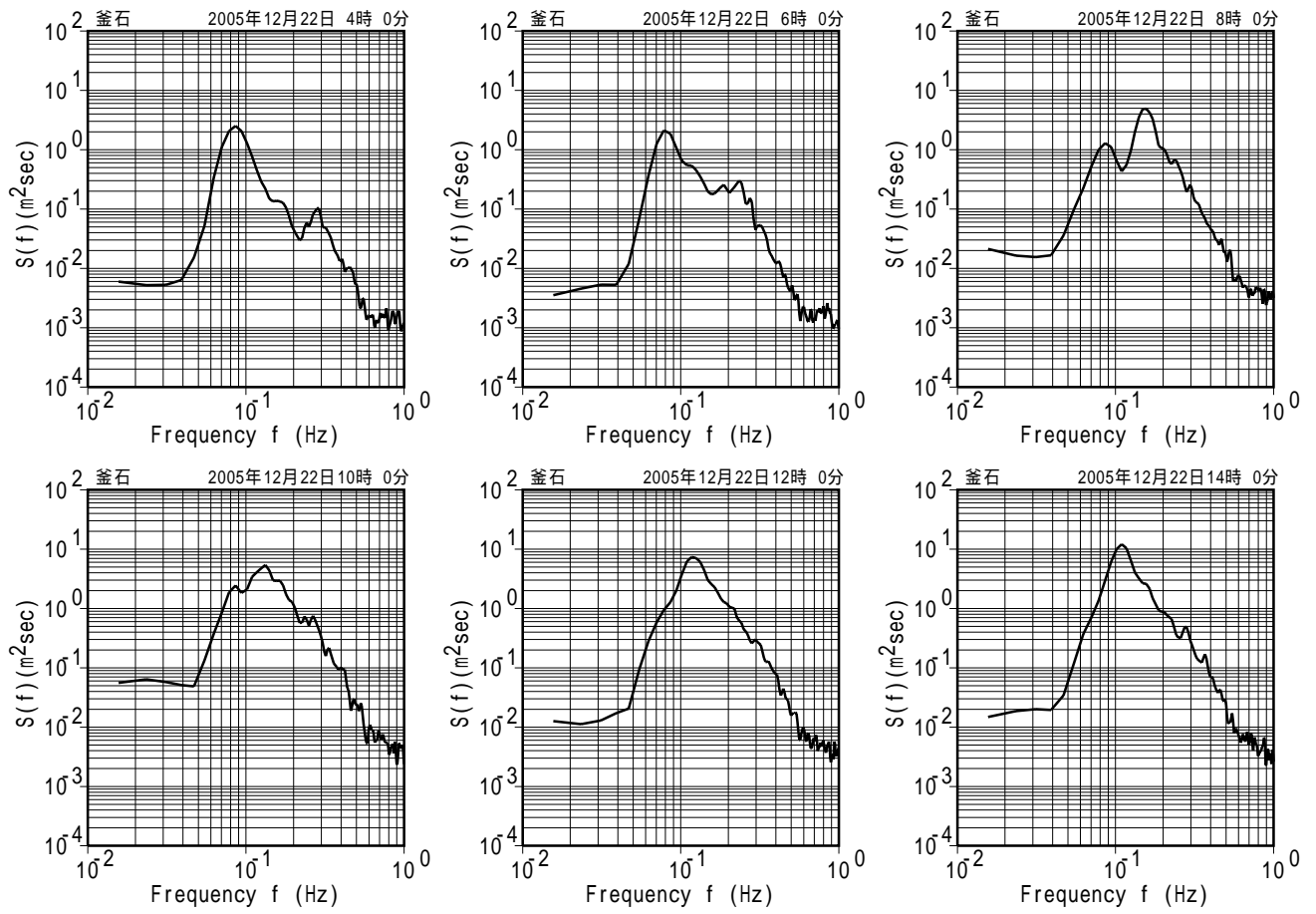
付図 - A.5.32 釜石 代表的な高波期間中のスペクトル
