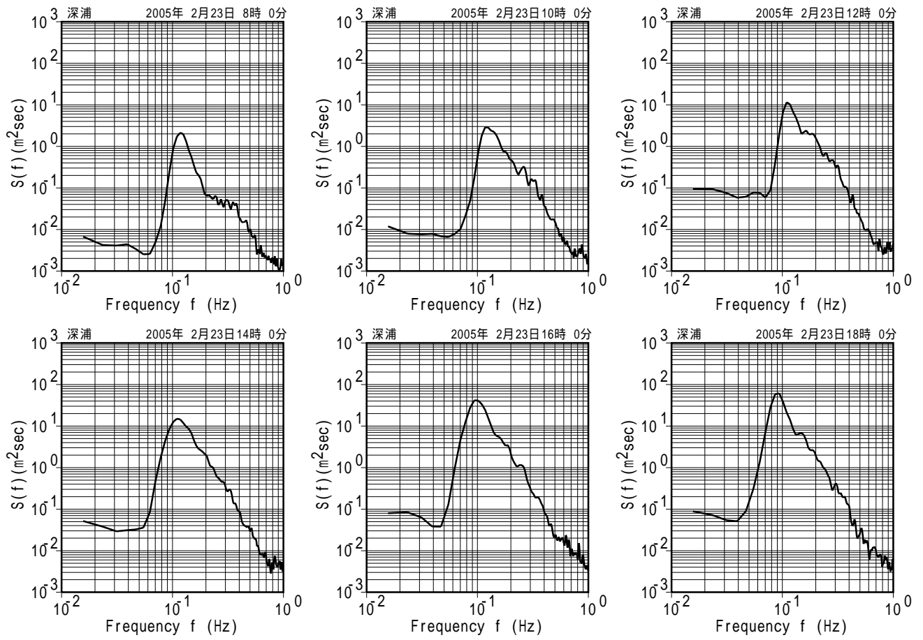
付図 - A.5.4 深浦 代表的な高波期間中のスペクトル
