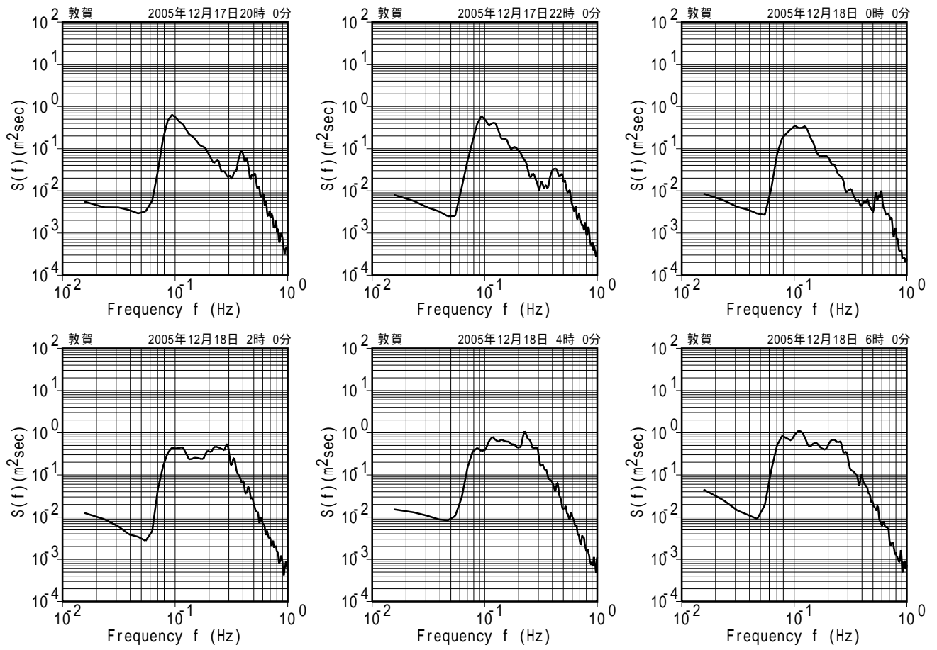
付図 - A.5.14 敦賀 代表的な高波期間中のスペクトル
