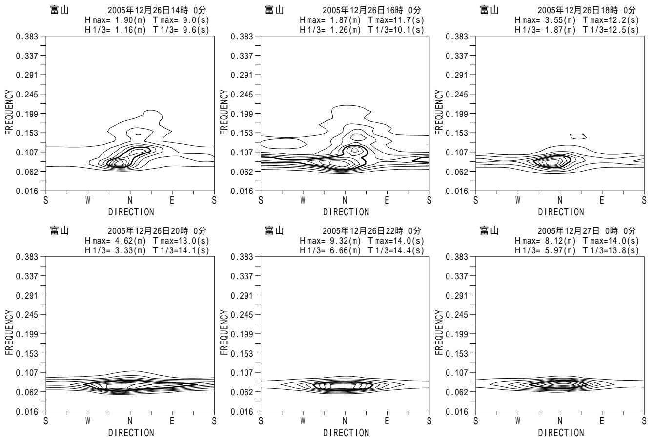
付図 - A.5.9 富山 代表的な高波期間中の方向スペクトル
