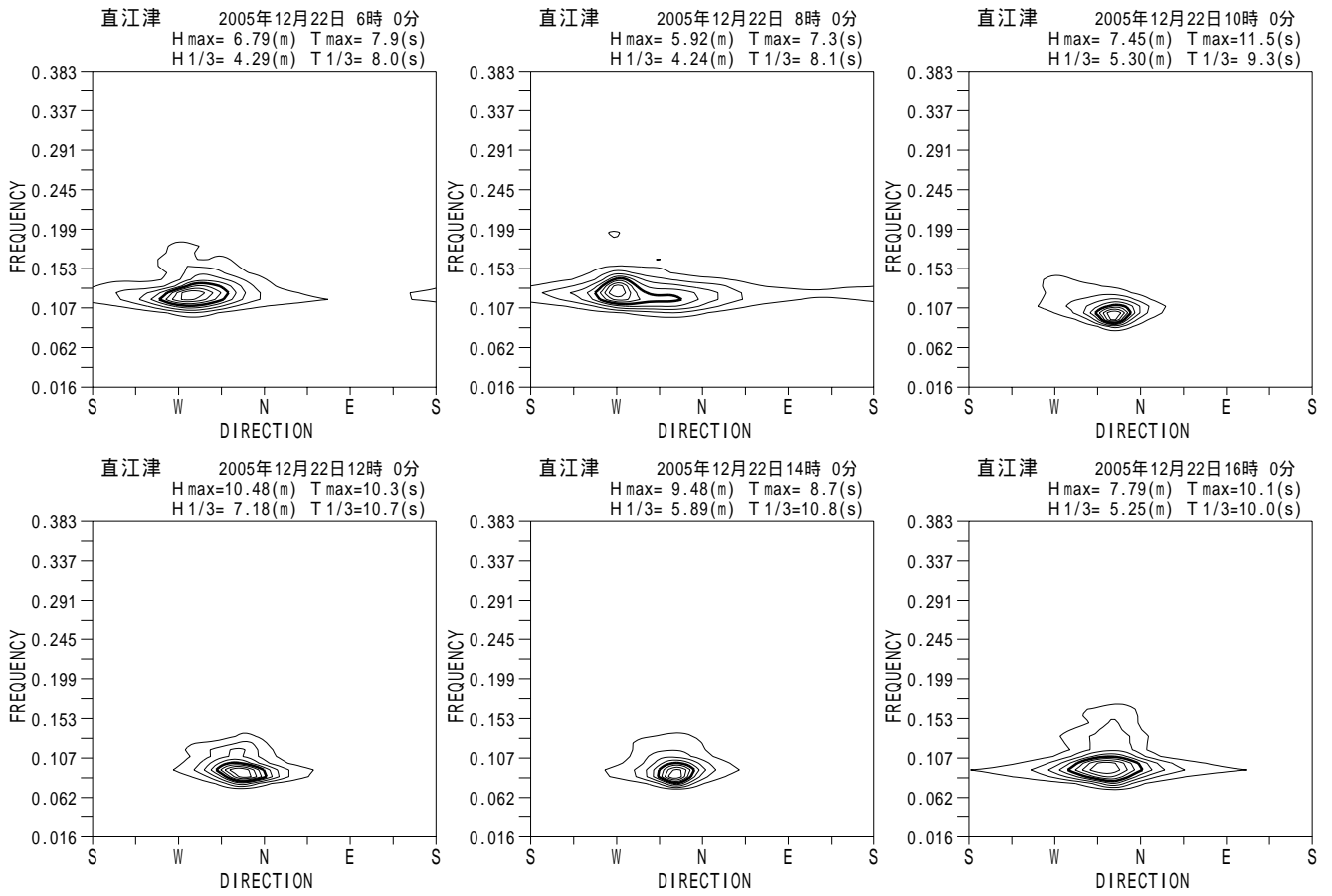
付図 - A.5.8 直江津 代表的な高波期間中の方向スペクトル
