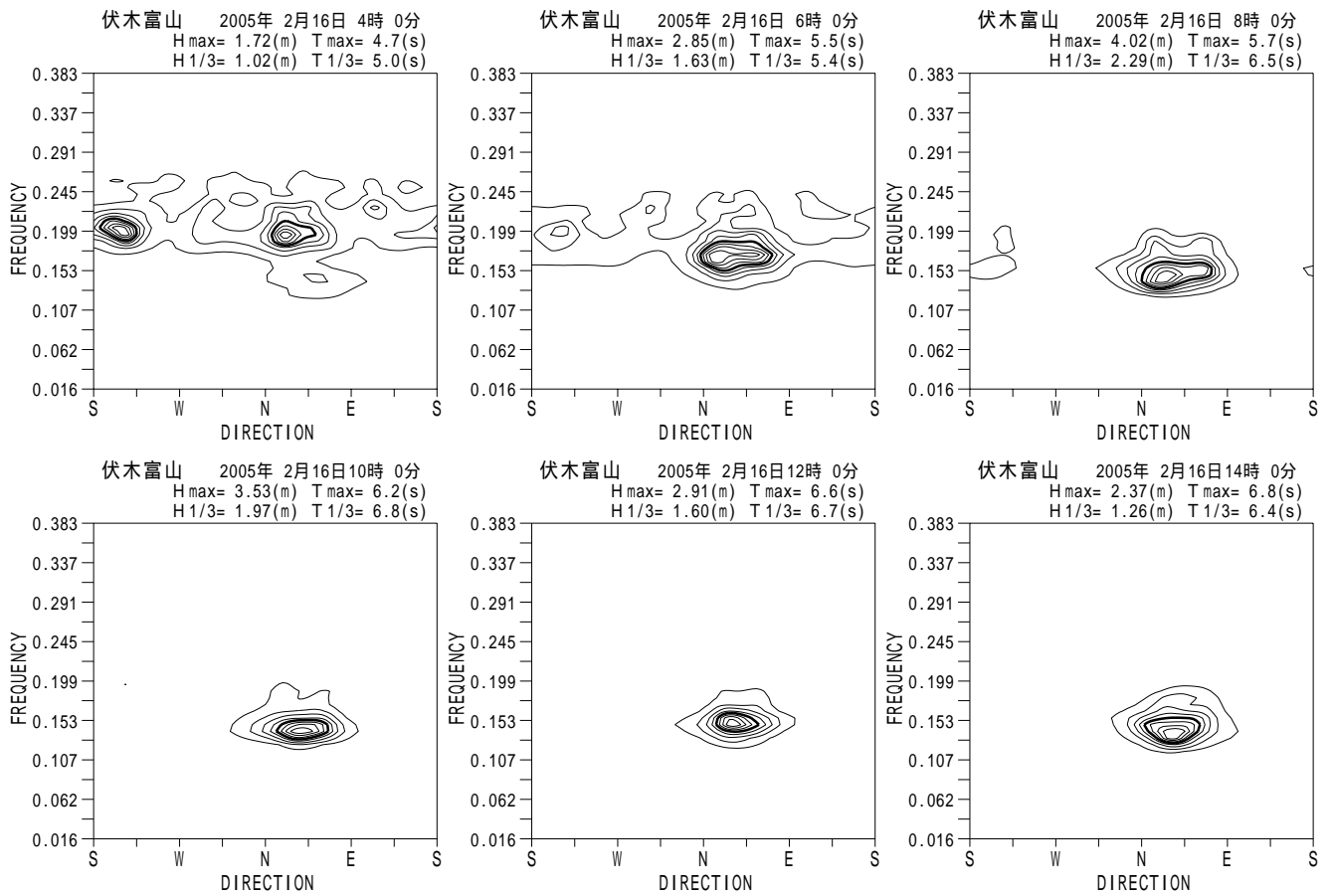
付図 - A.5.10 伏木富山 代表的な高波期間中の方向スペクトル
